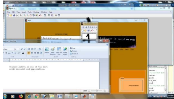
Fig8: Output
